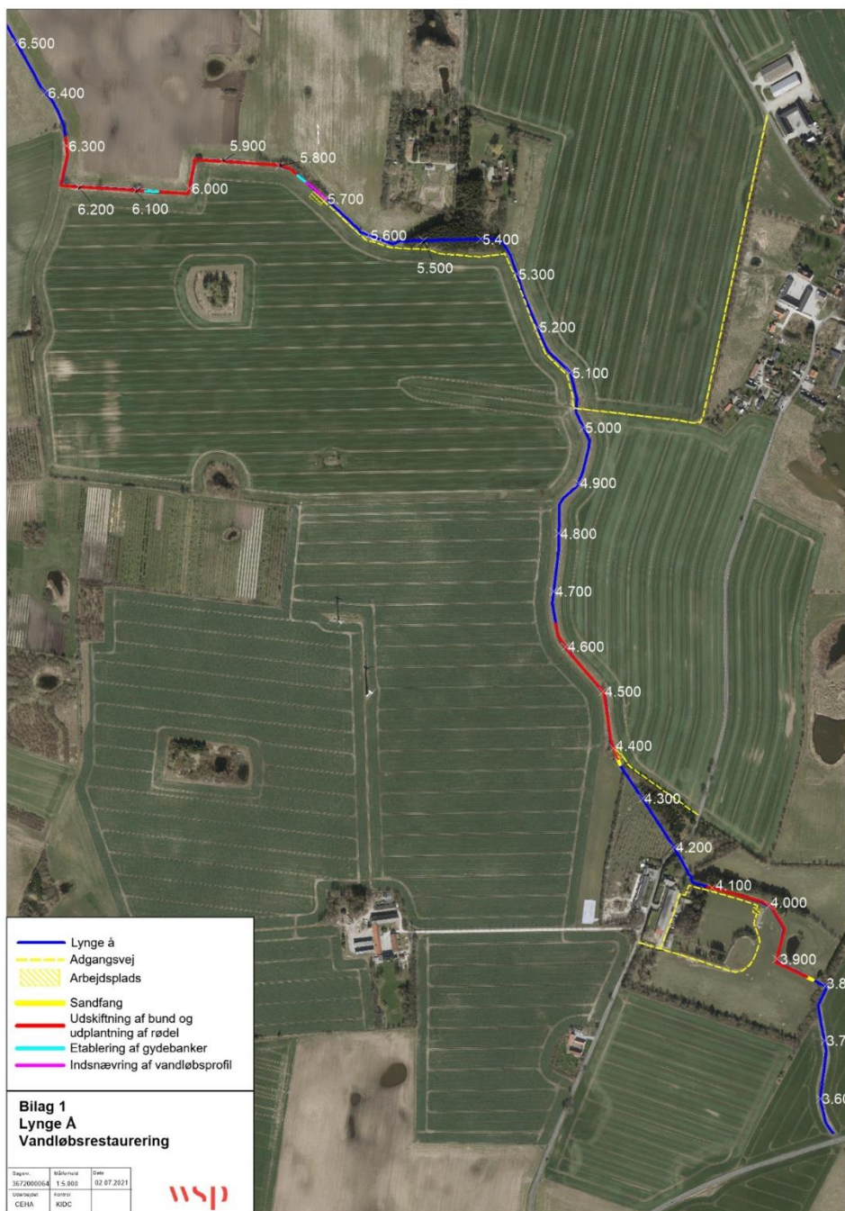
Figur 1 Oversigt over strækninger, hvor der direkte vil blive udført indsatser i vandløbet. Desuden foreslåede adgangsveje og arbejdsområder i anlægsperioden.
